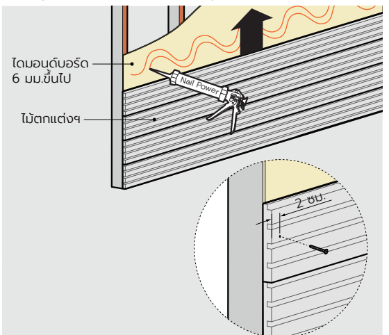
ตำแหน่งยึดสกรู ป้องกันการหลุด
