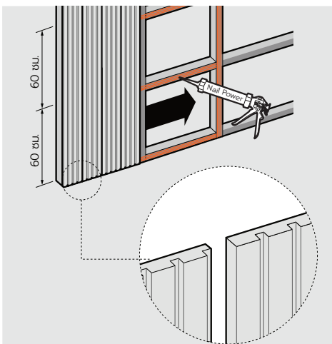
ลักษณะการต่อชนแนวตั้ง
