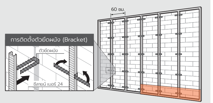
สำหรับผนังท้ออิฐ
